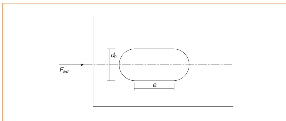
Figura 58.3. Agujeros rasgados
