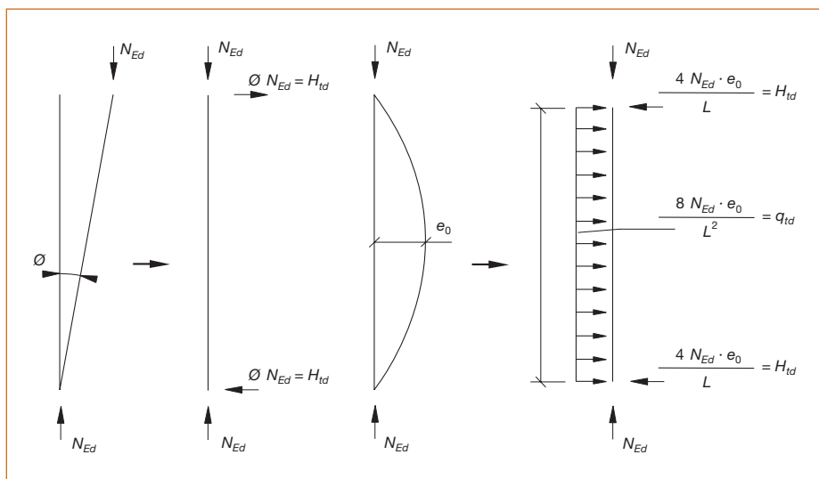
Figura 22.3.3.a. Fuerzas transversales equivalentes a las imperfecciones
