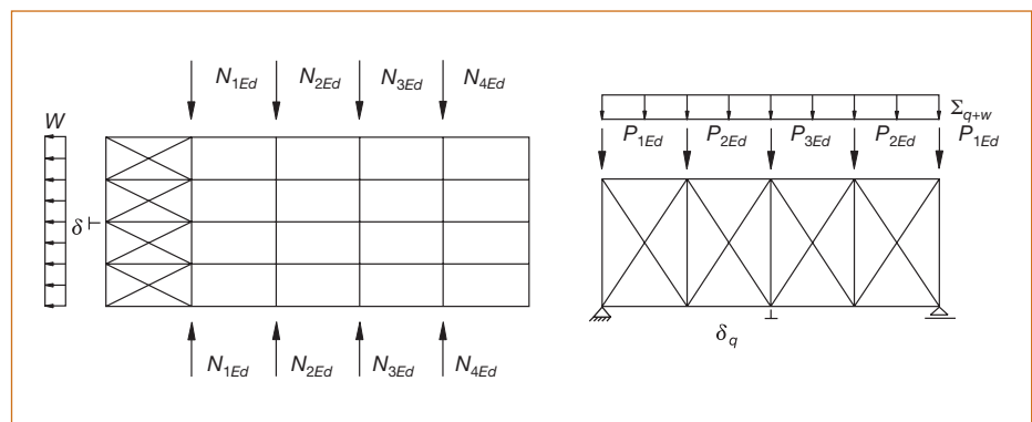
Figura 22.4.1.b. Fuerzas equivalentes incluyendo acciones exteriores
