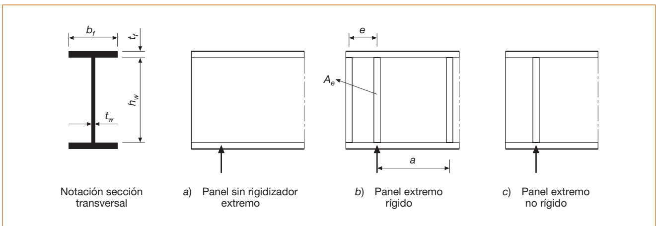
Figura 35.5.2. Criterio de clasificación del extremo del panel
