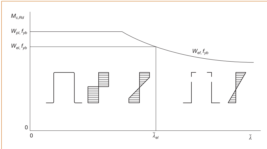
Figura 73.11.2. Resistencia de cálculo a flexión de secciones de clase 3
