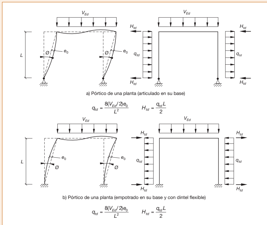
Figura 22.3.3.c. Fuerzas horizontales equivalentes adicionales por curvaturas iniciales en los elementos
