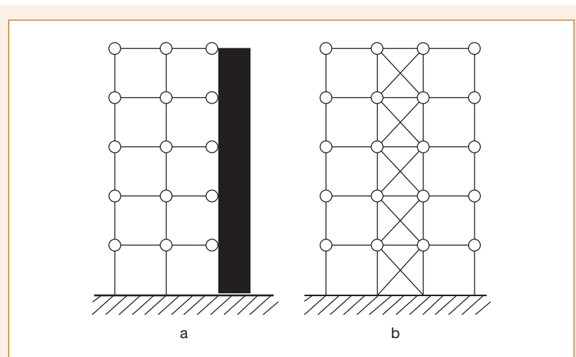
Figura 49 Arriostramientos de estructuras de acero: a) Mediante núcleos o pantallas de hormigón armado. b) Mediante elementos de acero
