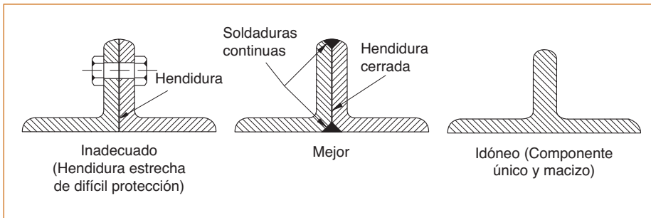
Figura 31.2.3.c. Tratamiento de huecos
