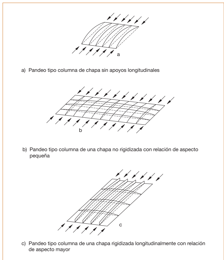
Figura A6.3. Pandeo tipo columna
