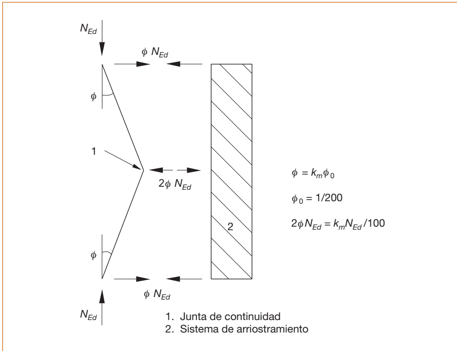
Figura 22.4.1.c. Fuerzas locales sobre el sistema de arriostramiento de elementos con junta de continuidad
