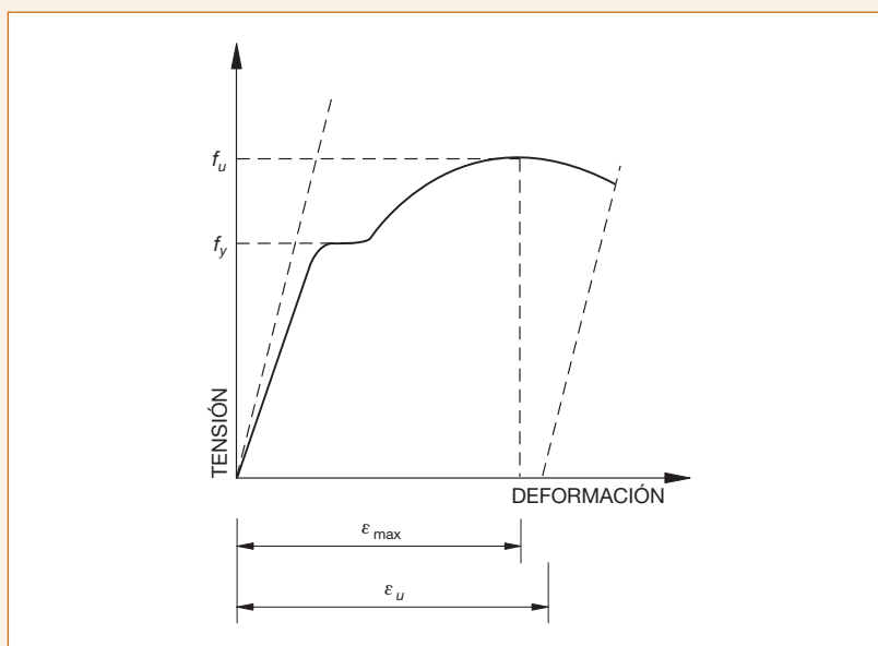
Figura 26.2. Diagrama tensión-deformación del acero
