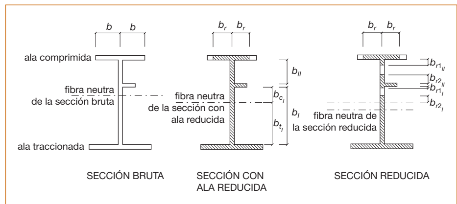
Figura 20.7.a. Sección reducida en secciones esbeltas rigidizadas
