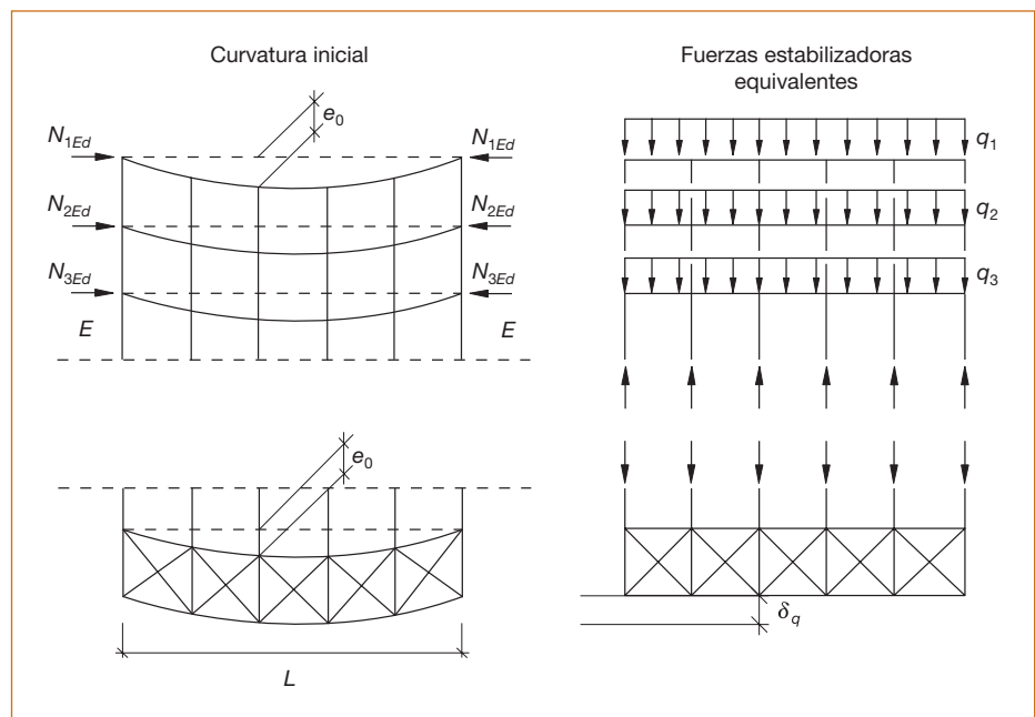
Figura 22.4.1.a. Imperfecciones sobre el sistema de arriostramiento
