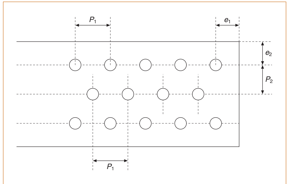
Figura 58.4.b. Agujeros al tresbolillo
