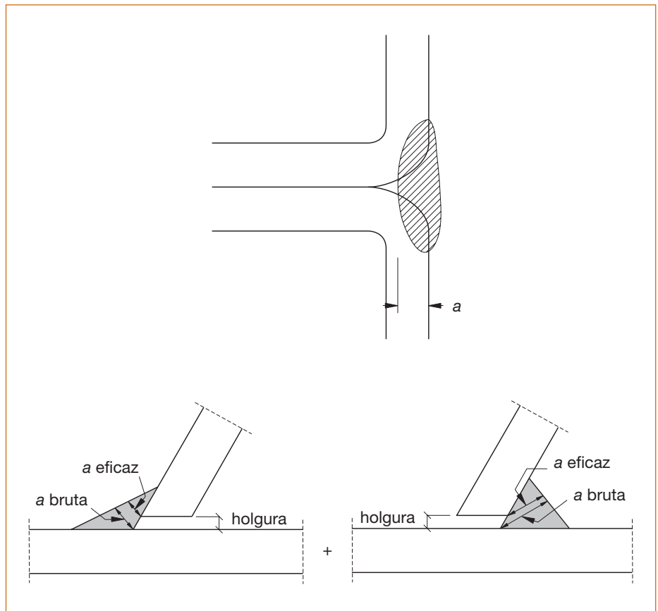
Figura 64.3.a. Gargantas eficaces en algunas uniones tubulares
