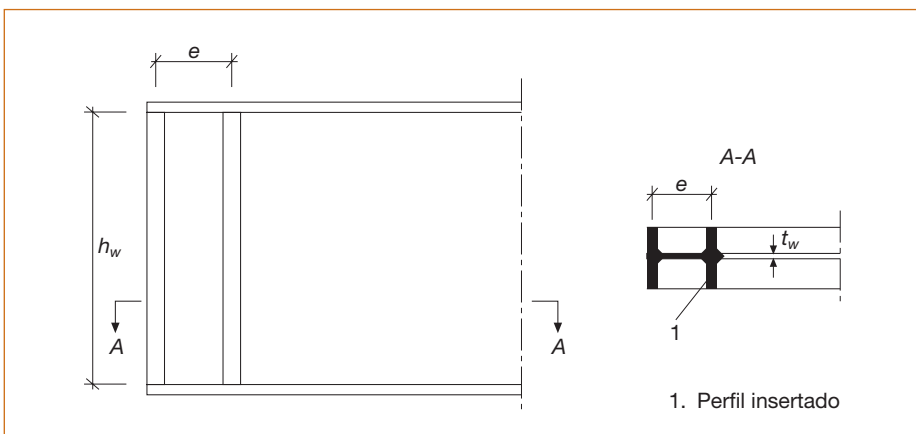
Figura 35.9.3.1. Perfil laminado formando un panel extremo rígido
