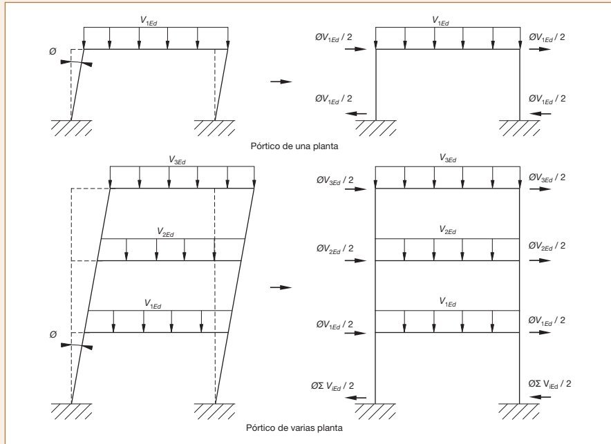
Figura 22.3.3.b. Fuerzas horizontales equivalentes a los defectos iniciales de verticalidad
