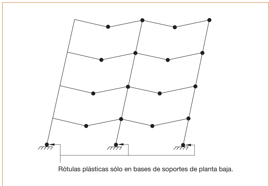
Figura 24.3. Mecanismo plástico incompleto en pórticos ortogonales de varias plantas
