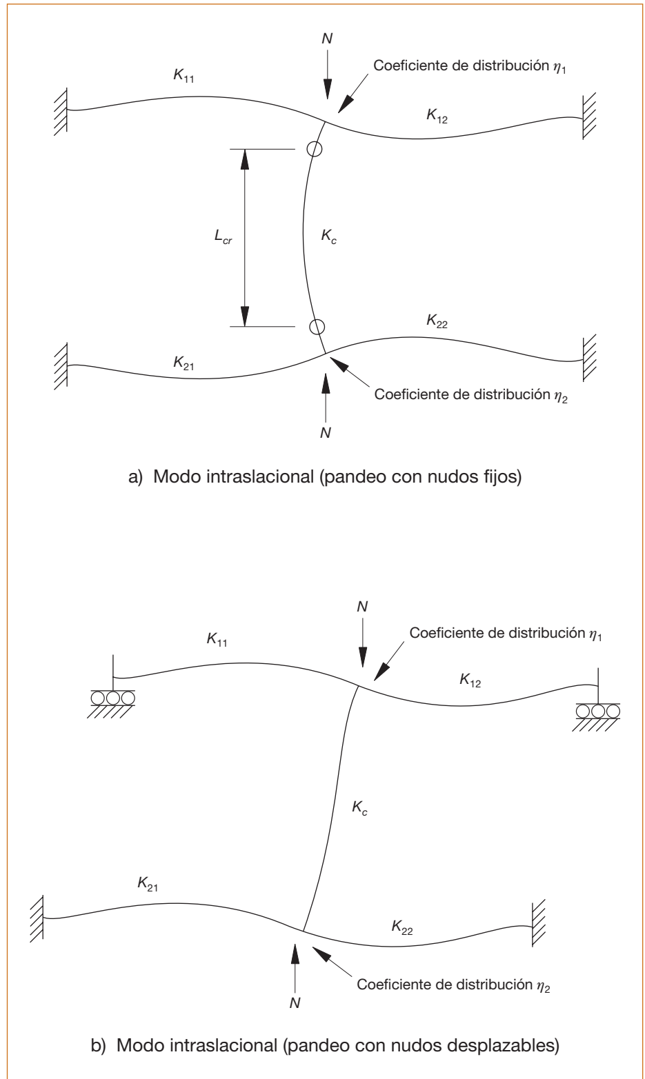
Figura A5.2.c. Coeficientes de distribución para soportes
