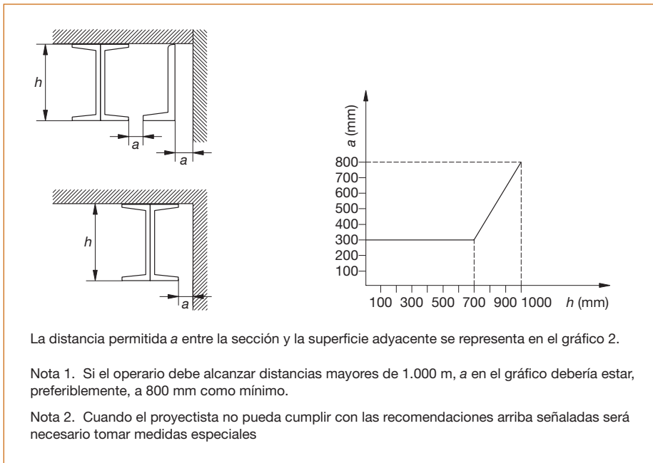
Figura 92.2.c. Distancias mínimas entre piezas cercanas (2)
