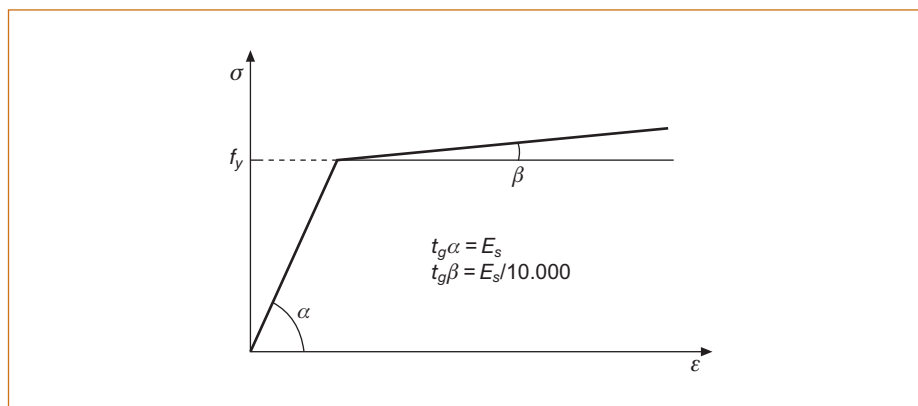
Figura 32.2.b Diagrama tensión-deformación bilineal, con segunda rama inclinada
