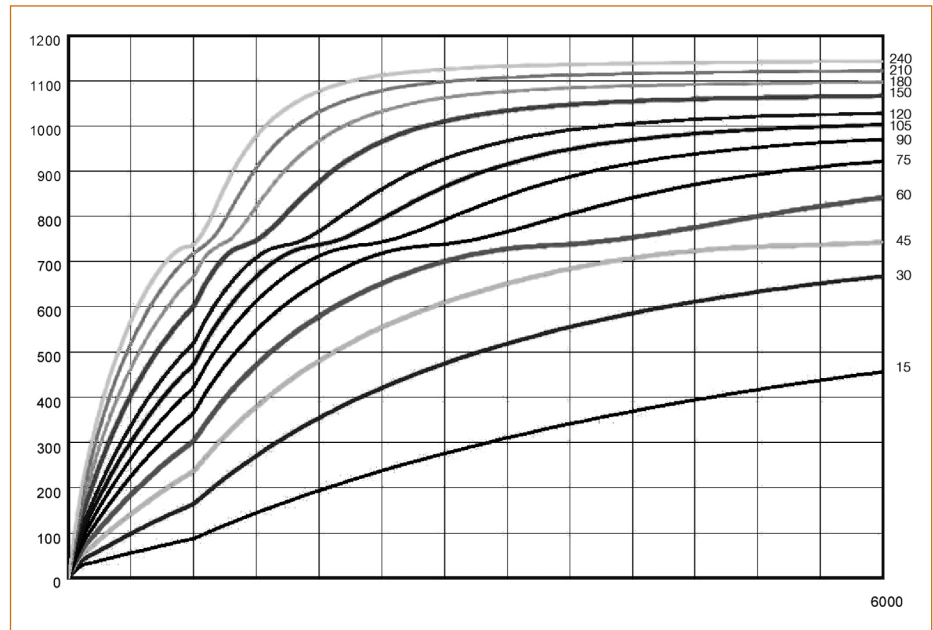
Figura 48.4.1 En ordenadas: temperaturas del acero \theta_a , 0 \leq \theta_a \leq 1.200 °C. En abscisas: variable s , 0 \leq s \leq 6\,000 W/(m^3 K) . Cada curva corresponde al valor indicado en t , en minutos
