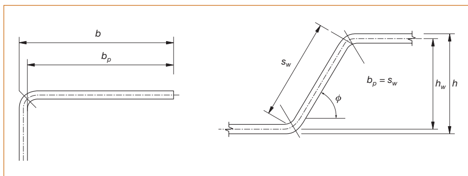
Figura 73.5. Anchura recta b_p
