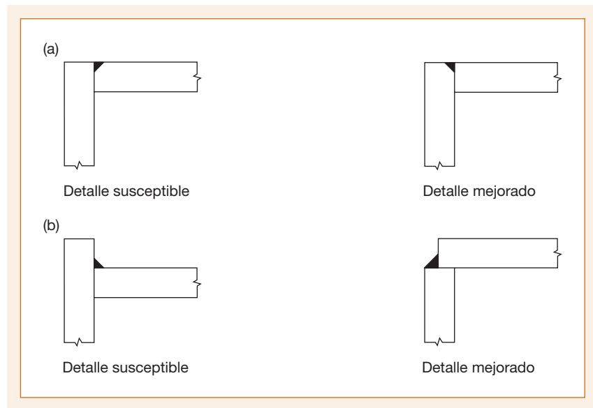
Figura 26.4. Mejora de detalles constructivos frente al desgarro laminar
