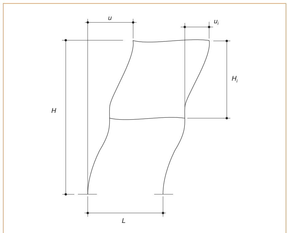
Figura 37.1.b. Definición de deformaciones horizontales
