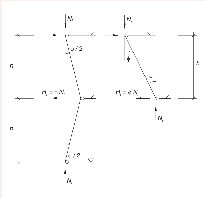
Figura 22.3.3.d. Esquema de fuerzas horizontales transmitidas por los soportes a los forjados
