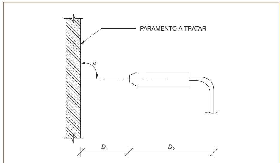
Figura 92.2.a. Disposición de las herramientas de mantenimiento
