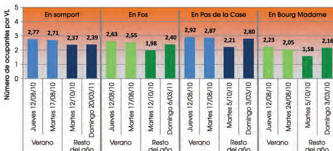
GRÁFICO 20. TASA DE OCUPACIÓN DE V.L. (ENCUESTA V.L. 2010 EN LOS PASOS CENTRALES)
