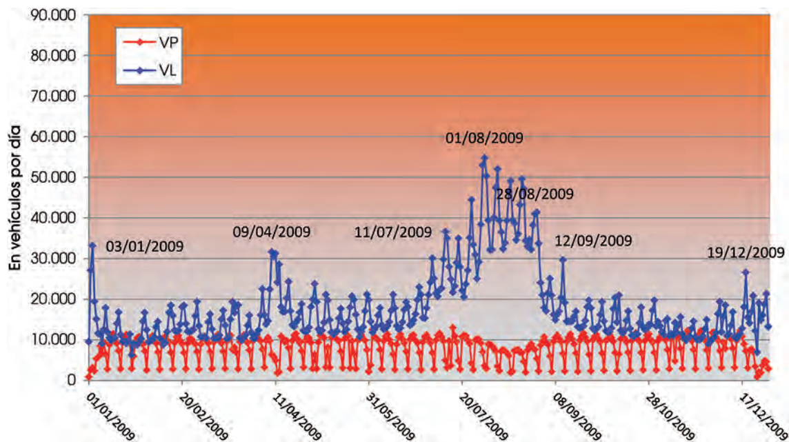
GRÁFICO 12. EVOLUCIÓN DIARIA DEL TRÁFICO EN LA AUTOPISTA A-63 EN 2009 (BIRIATOU)
