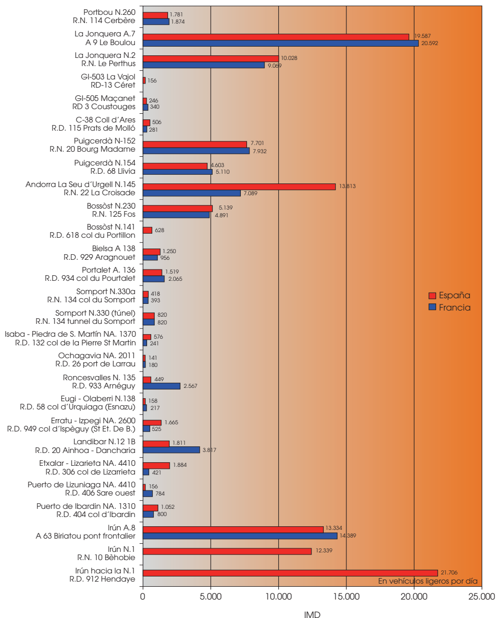
GRÁFICO 17. IMD ANUAL DE VEHÍCULOS LIGEROS EN LOS PUNTOS FRONTERIZOS EN EL AÑO 2009 (SUMA DE AMBOS SENTIDOS)
