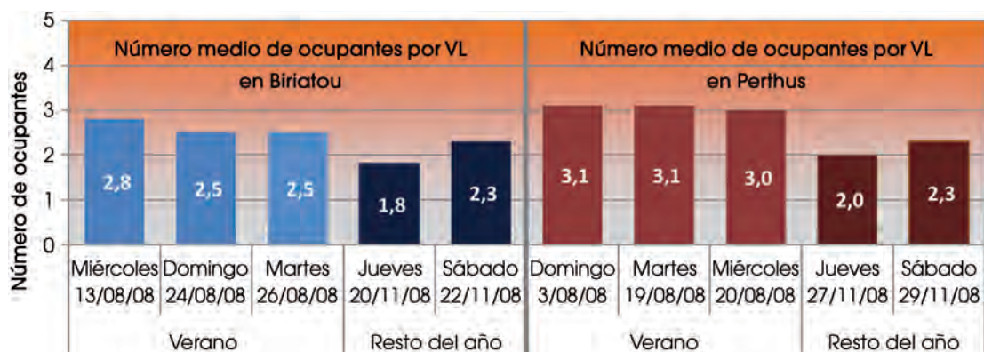
GRÁFICO 19. TASA DE OCUPACIÓN DE V.L. (ENCUESTA V.L. 2008 EN AUTOPISTAS)
