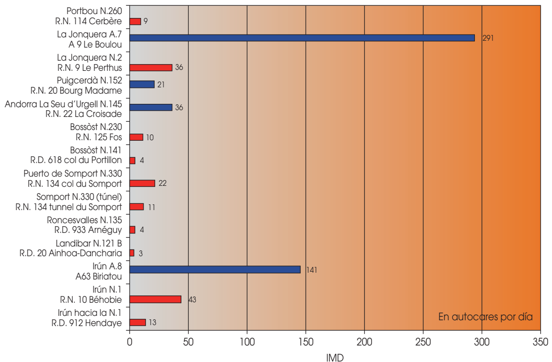
GRÁFICO 21. IMD ANUAL DE AUTOCARES EN LOS PUNTOS FRONTERIZOS EN EL AÑO 2009 (SUMA DE AMBOS SENTIDOS DE CIRCULACIÓN)
