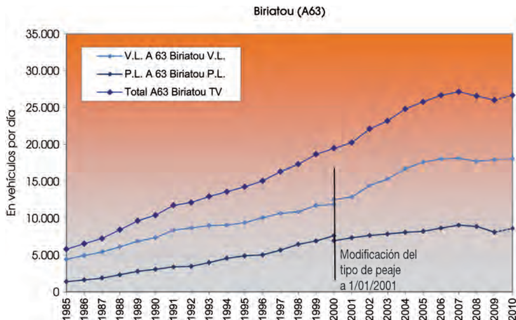
GRÁFICO 16. EVOLUCIÓN DEL TRÁFICO MEDIO ANUAL EN LAS DOS AUTOPISTAS
