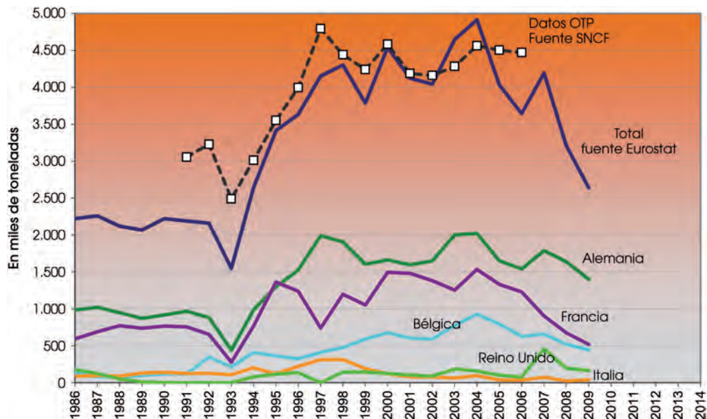
GRÁFICO 34. EVOLUCIÓN DEL TRÁFICO FERROVIARIO DE MERCANCÍAS EN AMBOS SENTIDOS A TRAVÉS DE LOS PIRINEOS (EN MILES DE TONELADAS)
