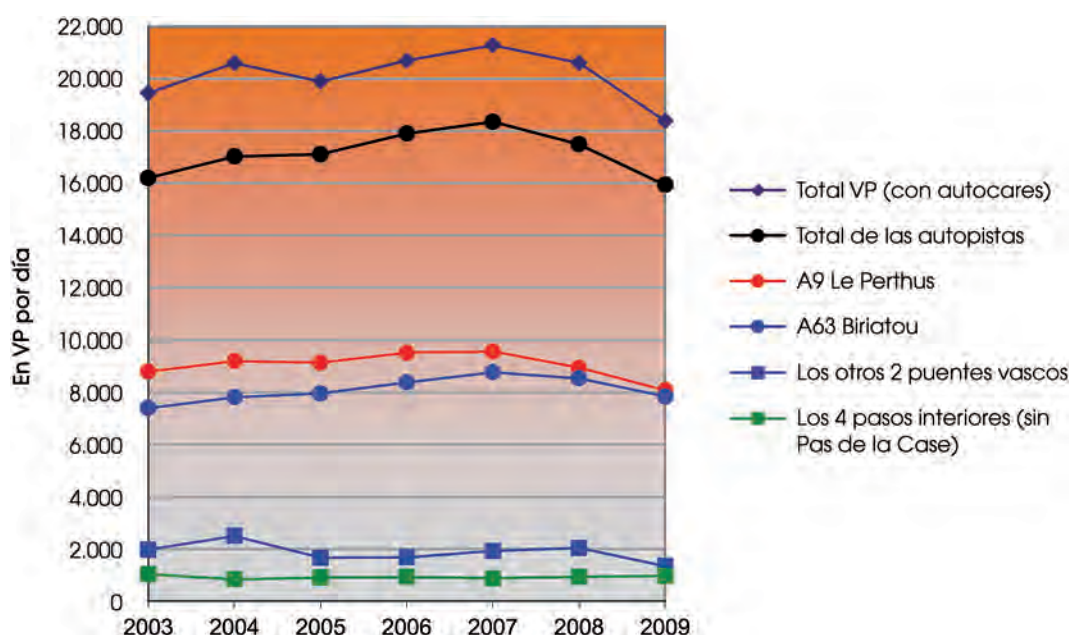
GRÁFICO 31. EVOLUCIÓN DE LA IMD ANUAL DE LOS V.P., QUE CRUZAN LA FRONTERA FRANCO-ESPAÑOLA
