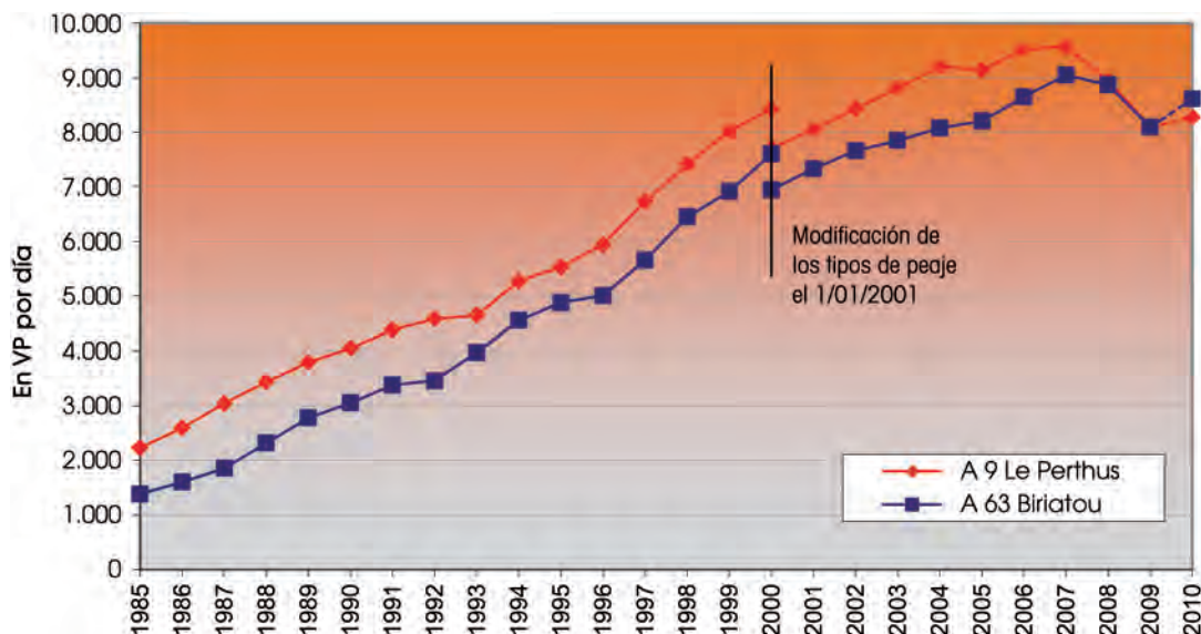
GRÁFICO 33. EVOLUCIÓN DE LA IMD ANUAL DE VEHÍCULOS PESADOS EN LAS 2 AUTOPISTAS (1985-2009)
