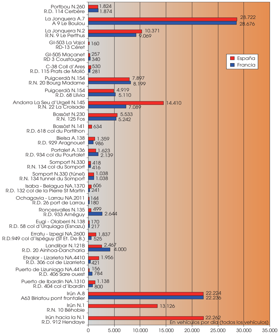
GRÁFICO 11. IMD ANUAL EN LOS PUNTOS FRONTERIZOS EN EL AÑO 2009 (TODOS LOS VEHÍCULOS)
