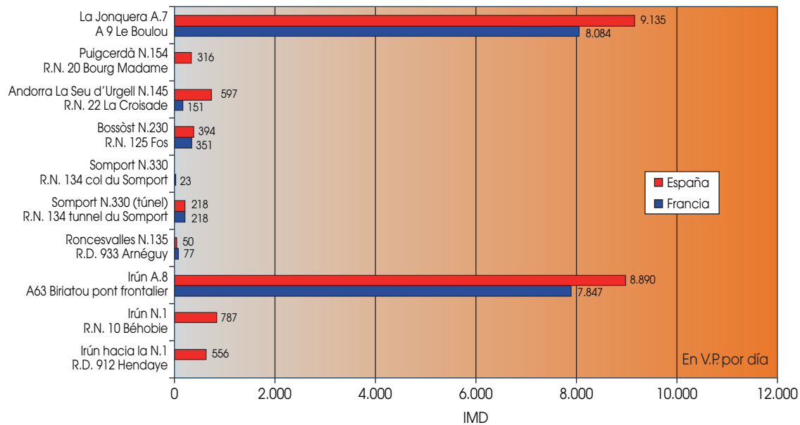
GRÁFICO 29. IMD VEHÍCULOS PESADOS EN LOS PUNTOS FRONTERIZOS DE MAYOR TRÁFICO
