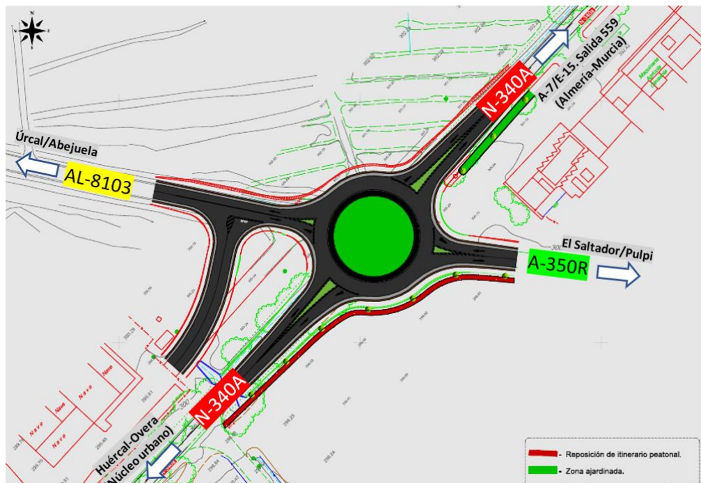
Detalle de la glorieta propuesta
